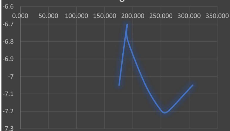
Curva NU Ori Mag. vs Día Juliano
