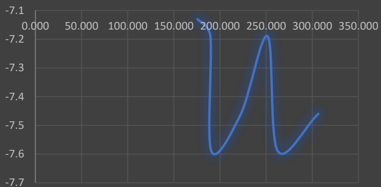
Curva KX Orion - Mag. vs Día Juliano
