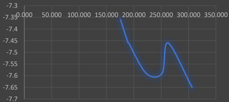
Curva V359 Ori - Mag. vs Día Juliano
